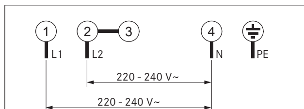
рис. 6.38 Схема подключения, 2-фазное подключение
