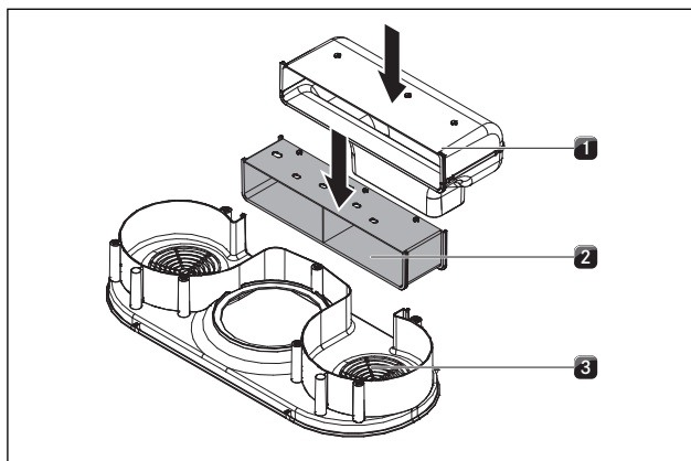
рис. 6.31 Установка удлинителя канала отвода воздуха
