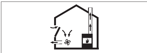
рис. 6.21 Монтаж отвода воздуха - правильно
