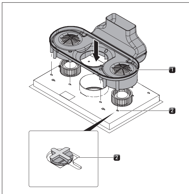
рис. 6.32 Установка узла воздуховода на основании варочной панели
