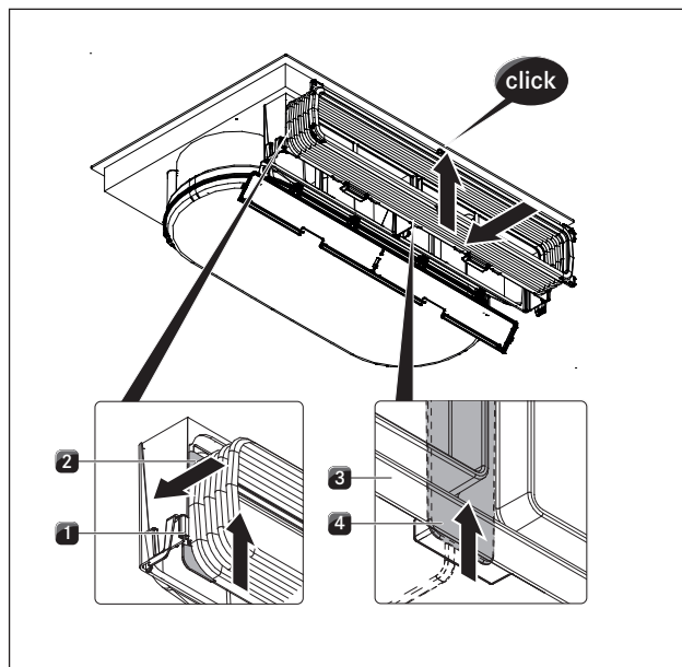
рис. 6.17 Установка рамки эластичного канала
