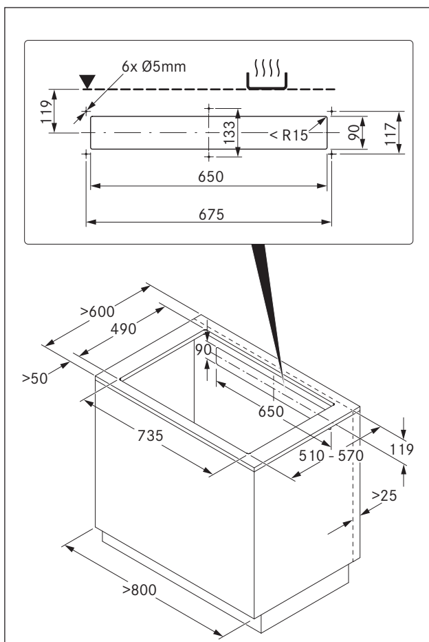
рис. 6.11 Размеры мебели для модели с циркуляцией воздуха
