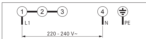
рис. 6.39 Схема подключения, 1-фазное подключение
