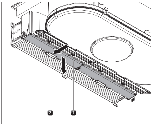
рис. 8.8 Достаньте фильтры с активированным углем
