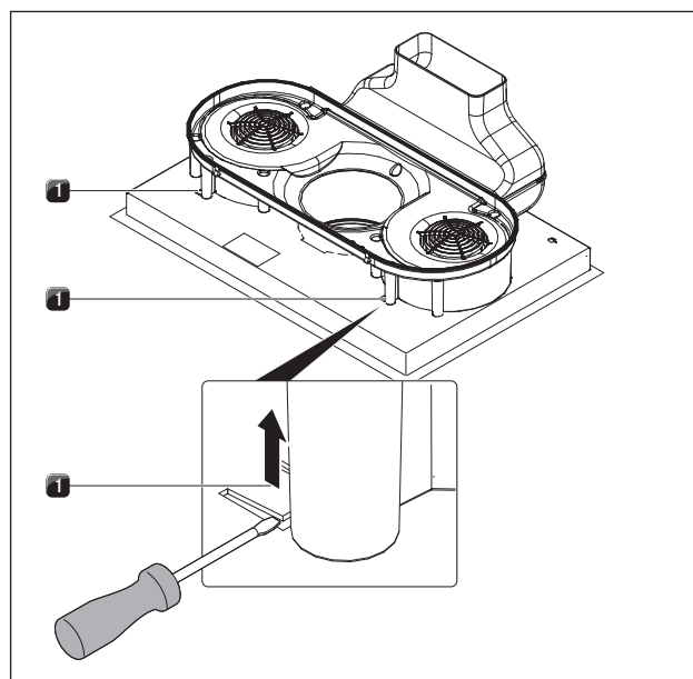
рис. 6.34 Фиксатор положения
