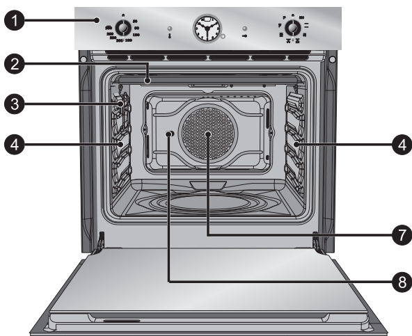
Пиролитическая модель
