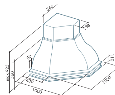
angolo/wall corner
